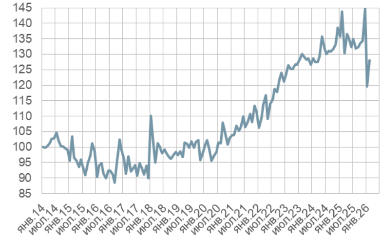
Строительство (янв. 2014 = 100)
